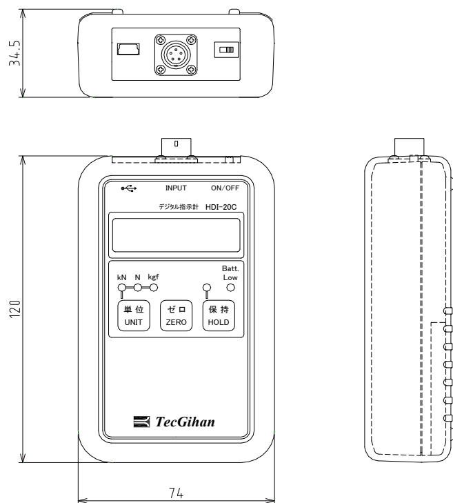
リニアライズ機能付デジタル指示計 外観図
