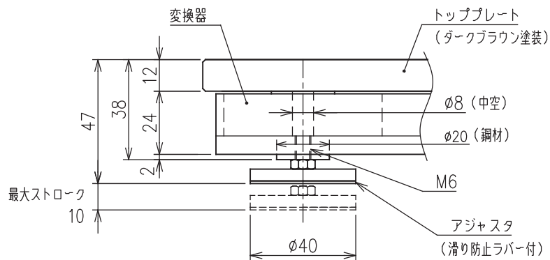
A拡大図
